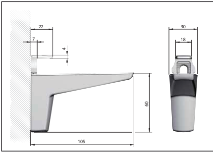
Shelf Dimensions
